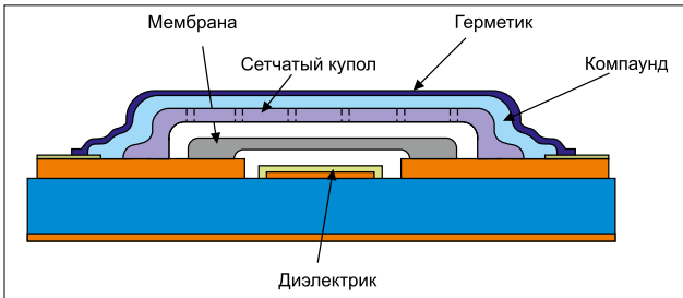
▲ Рис. 5. Герметизация МЭМС защитным куполом
