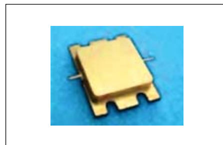
Рис. 4. Согласованный 55-Вт транзистор CHZ050A-SEA компании United Monolithic Semiconductors
