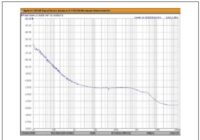
Рис. 4. Синтезатор частоты QuickSyn демонстрирует фазовые шумы ниже –120 дБн/Гц при 10-Гц отстройке от выходной частоты 10 ГГц
